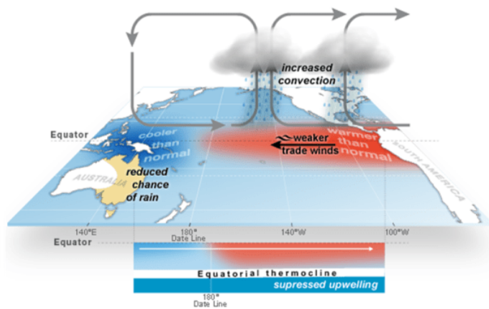
El Niño–Southern Oscillation (ENSO): El Niño
